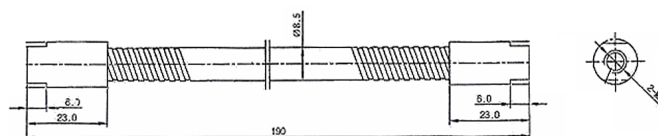
金屬軟管尺寸圖P-2
